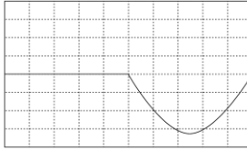
ARB7 サイン波 全波整流 正極
